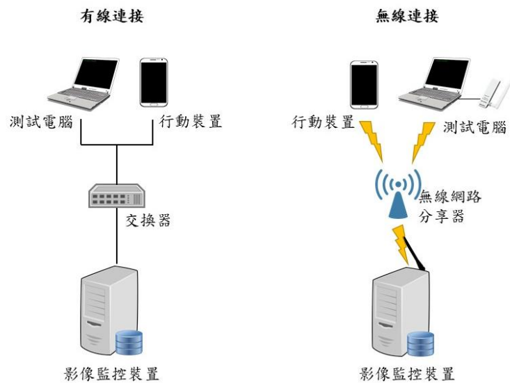
圖 5 測試示意圖
